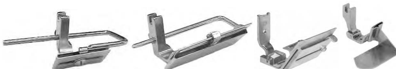
A706BIS pedino con tubo guida nastro regolabile tubi intercambiabili in dotazione A706 pedino guida nastro regolabile tubo grande fisso S570G guida nastro regolabile per ZZ attacco piatto A689G guida nastro mm 12,7 con appoggio (S532)
